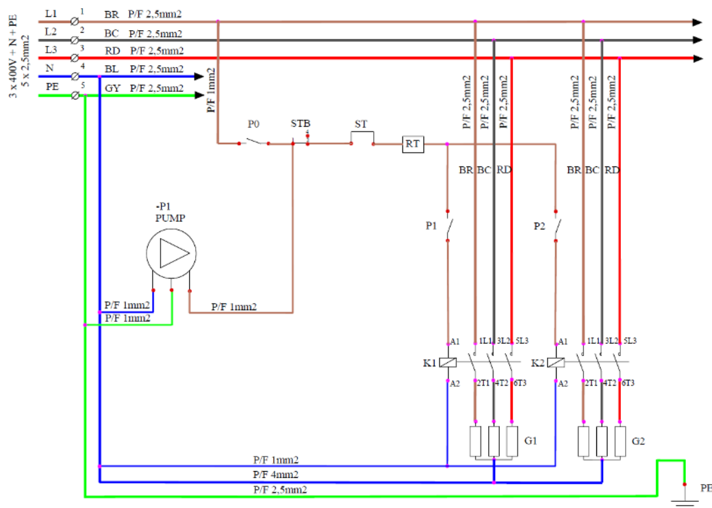
Slika 9. Šema povezivanja EK Classic 12 kW UGRADNI, EK Classic 18 kW UGRADNI
