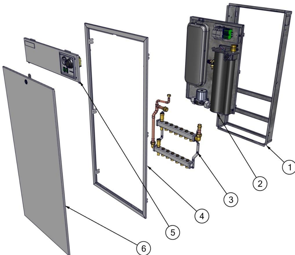
Slika 5. Redosled za montažu kotla u zid
