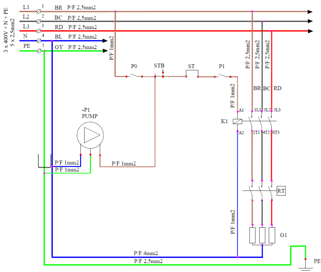
Slika 8. Šema povezivanja EK Classic 06 kW UGRADNI, EK Classic 09 kW UGRADNI
