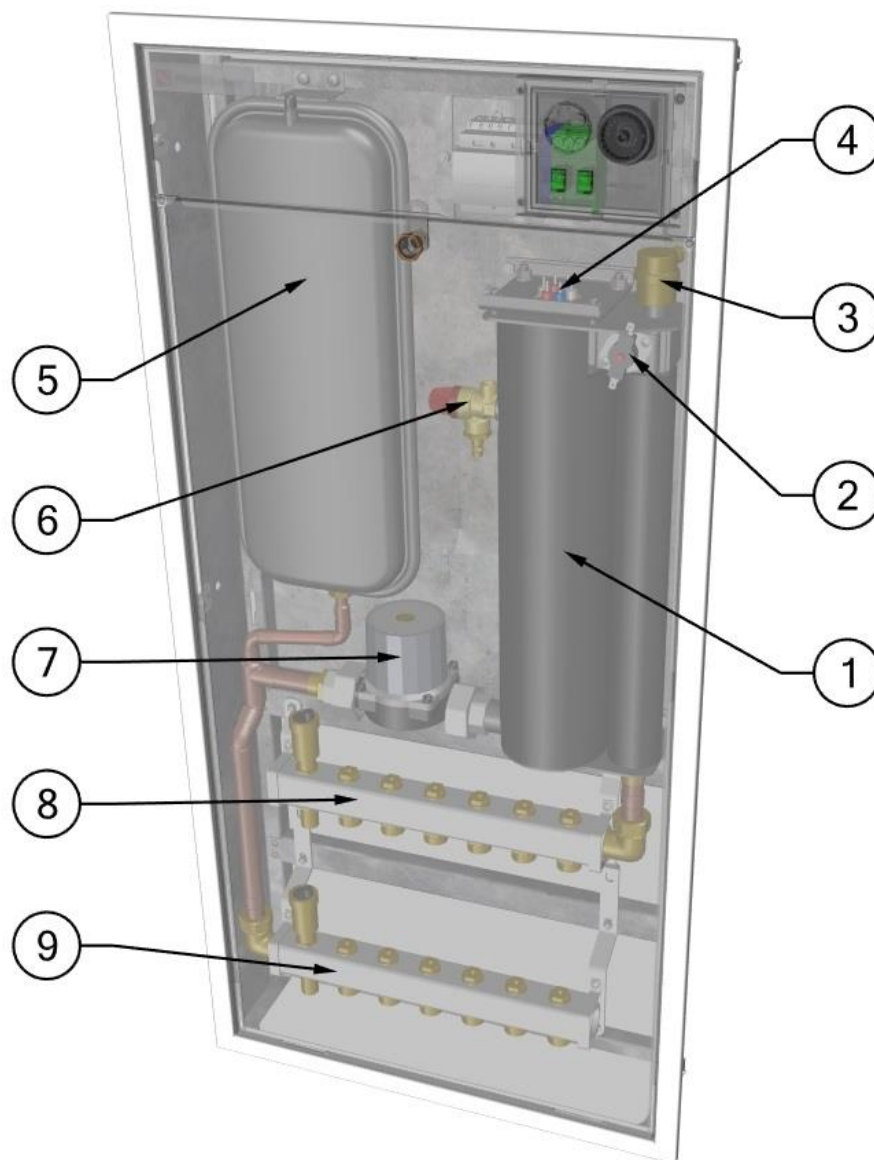
Slika 2. Komponente kotla
